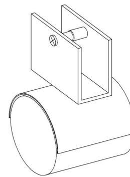
Ролик опорный крепится на межсекционную стяжку L=16мм
