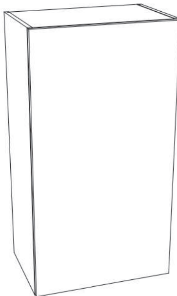
Мария МШН 60.96 Шкаф навесной Размеры (ВхШхГ) 965х600х336
