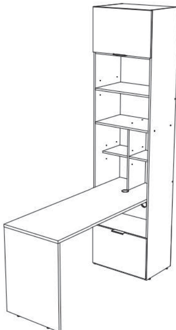
Мария МСС 60.120 Стеллаж-стол артикул Ж.01.03.01.02 Размеры (ВхШхГ) 2400х1603х600
