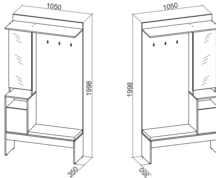
Левая сборка
