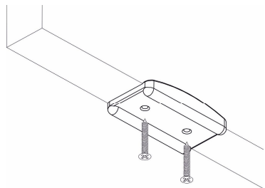
Установка подпятника
