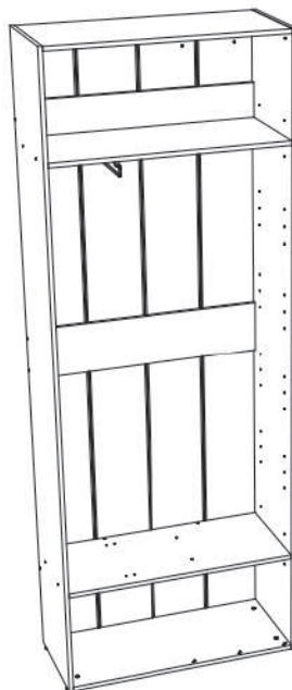
Мария МШ / МШУ 90.40 Шкаф артикул Ж.01.01.01.02 Размеры (ВхШхГ) 2400х900х403
