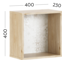
Мод. 7 Модуль навесной
