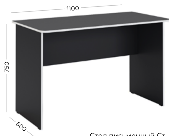
Стол письменный Ст-3
