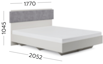
МКК 1,6 Кровать на 1600
