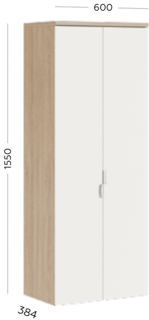
Мод.5 Шкаф Комплектуется только с мод.6 или мод.7
