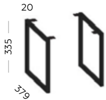
МТК 60 / МТК 90 / МТК 120 Опоры для консоли
