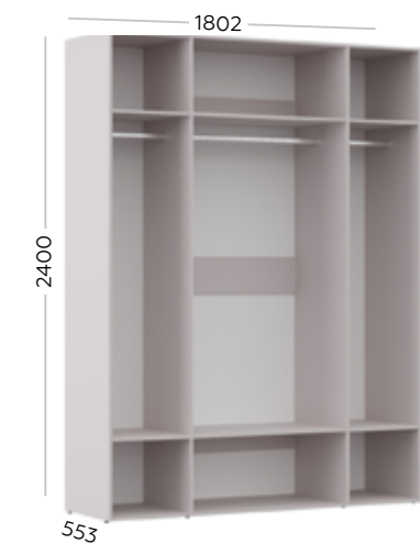
МШ 180.55 КОРПУС Шкаф
