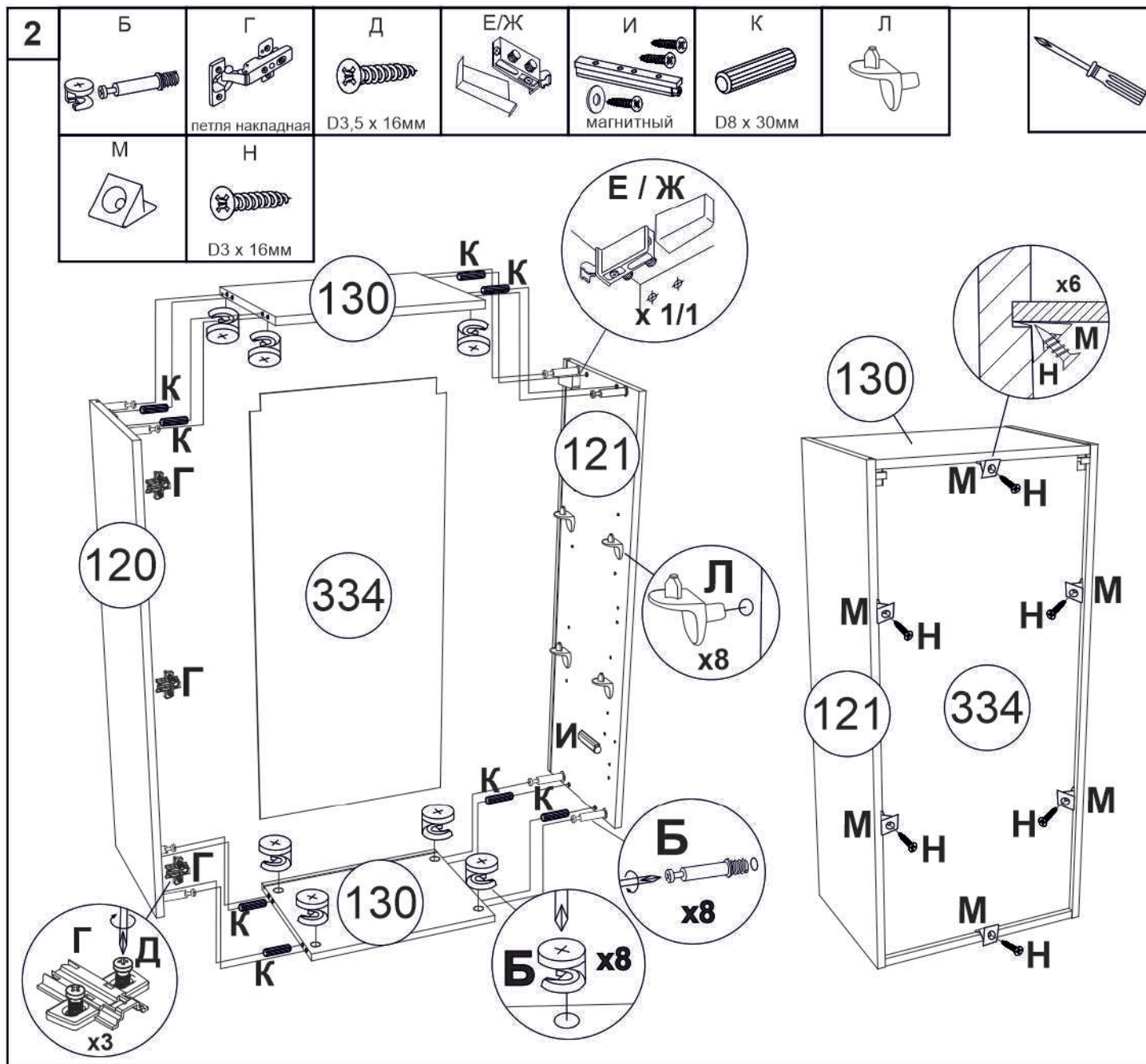
Схема установки механизма Push to open
