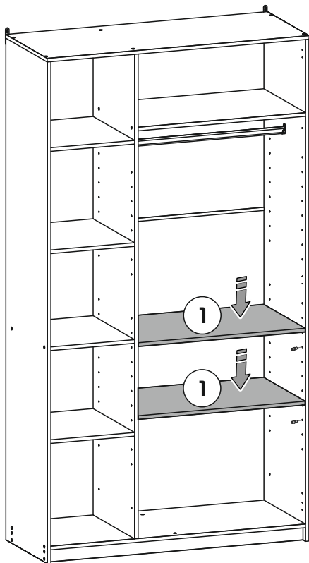
Шкаф 3-х створчатый с доводчиками Мод 120 см ЛДСП
