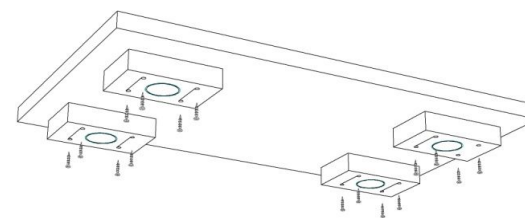
Установка опоры
