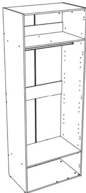
Мария МШ / МШУ 90.55 Шкаф артикул Ж.01.01.01.02 Размеры (ВхШхГ) 2400х900х553
