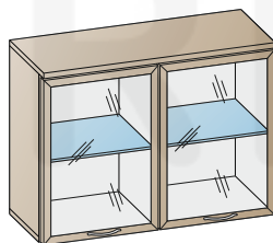
АН-1036 742x1080x352
