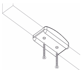
Установка подпятника
