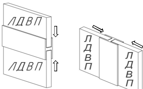
Соединение ЛДВП стыковочным брусом
