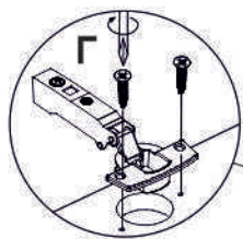
петля накладная
