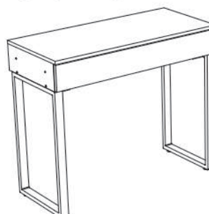
Мария МТ 90 Тумба + Мария Опоры для стола МТС 90 / МТС 120 Размеры (ВхШхГ) 765x901x418
