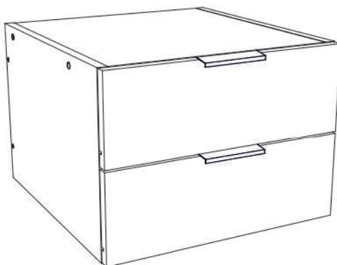
Мария Тумба подвесная артикул Ж.01.02.06.00 Размеры (ВхШхГ) 285x400x416
