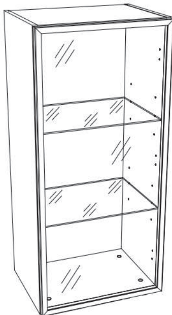
Мария МШН 45.96V Шкаф навесной витрина Размеры (ВхШхГ) 965x450x340
